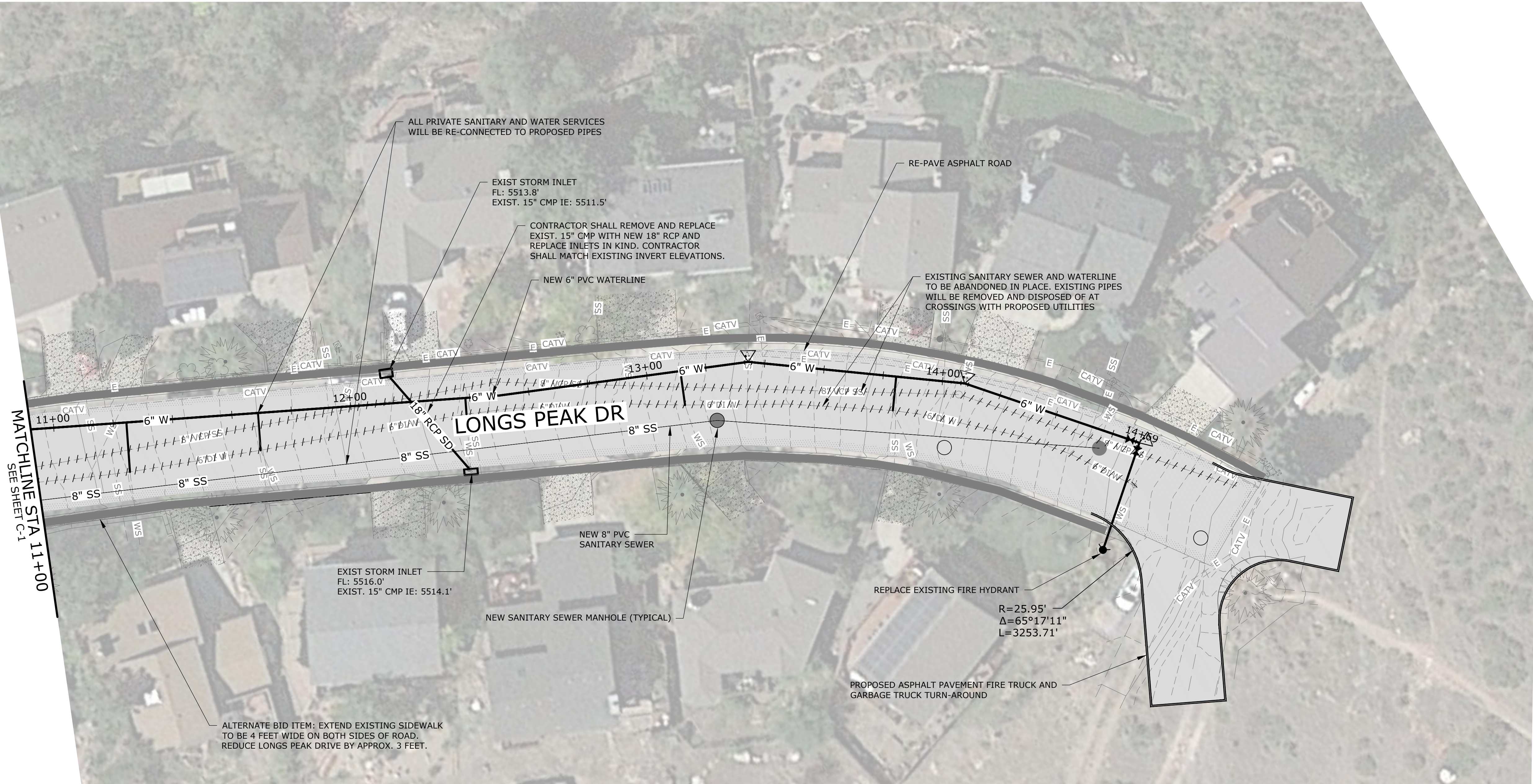
PLAN SCALE: 1"=20'
